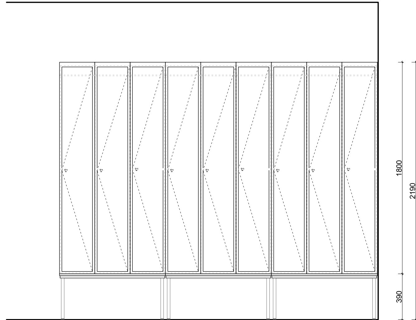
POHLED_1 ČELNÍ 1:20 @ A1
