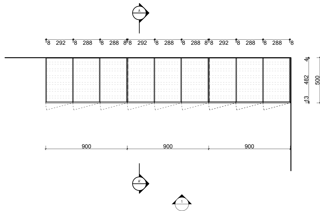
PŮDORYS HORIZONTÁLNÍ ŘEZ 1:20 @ A1
