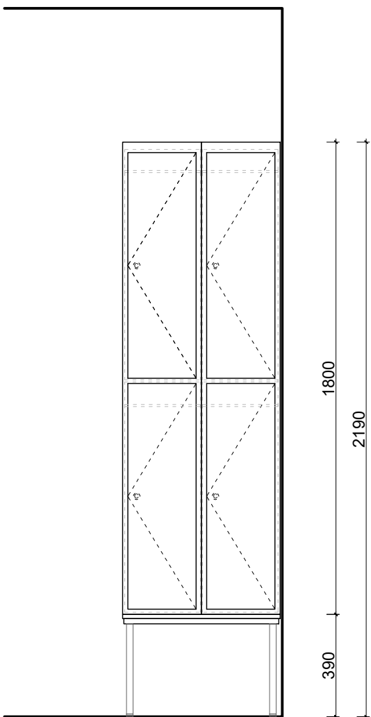
POHLED_1 ČELNÍ 1:20 @ A2
