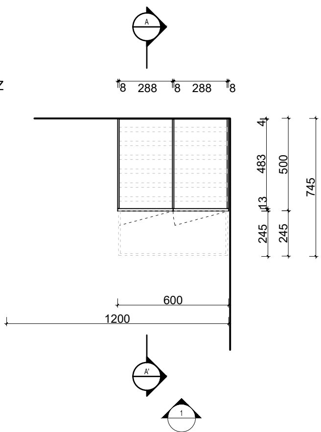
PŮDORYS HORIZONTÁLNÍ ŘEZ 1:20 @ A2
