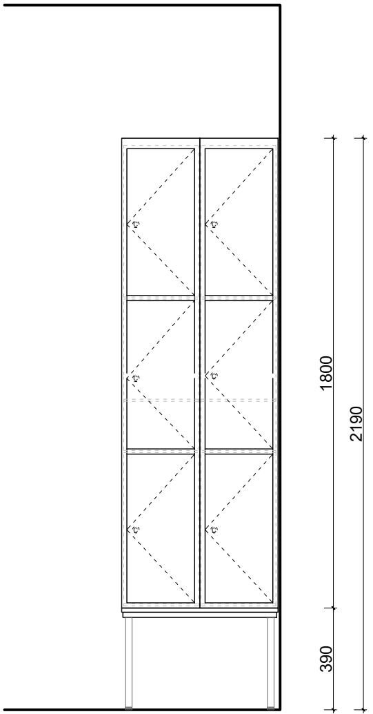
POHLED_1 ČELNÍ 1:20 @ A1
