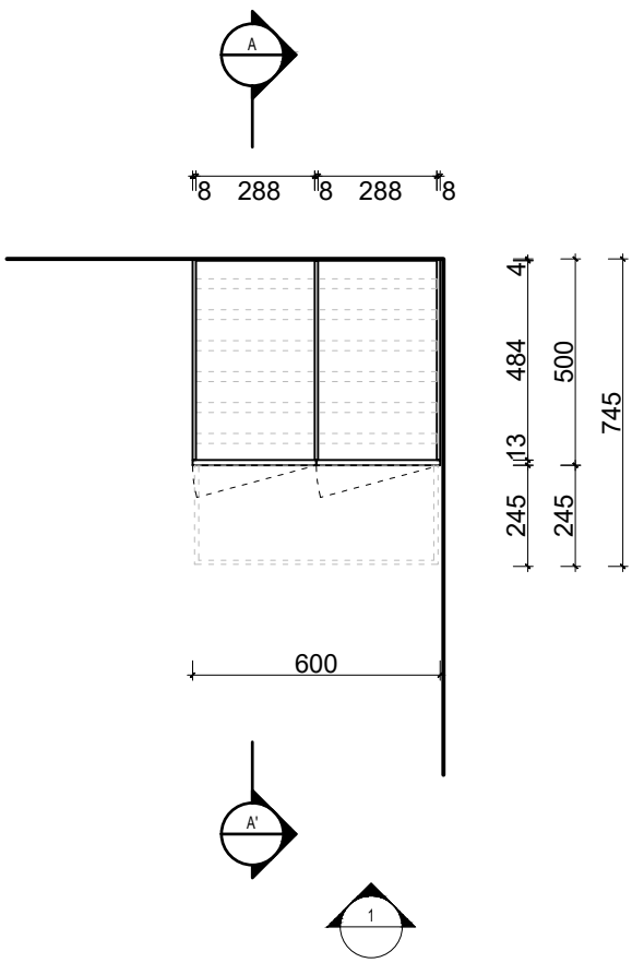
PŮDORYS HORIZONTÁLNÍ ŘEZ 1:20 @ A1
