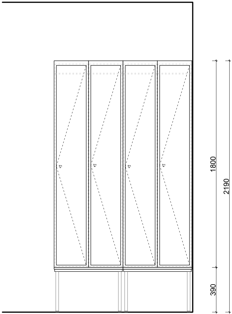
POHLED_1 ČELNÍ 1:20 @ A1
