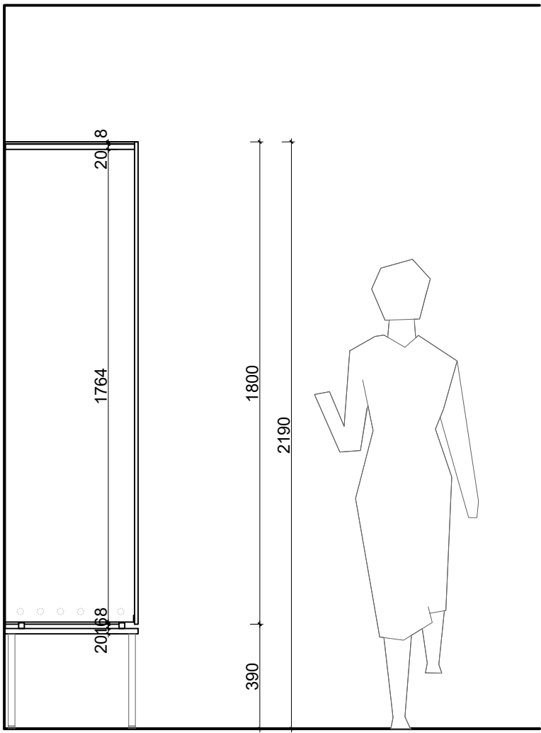
ŘEZ A-A 1:20 @ A1
