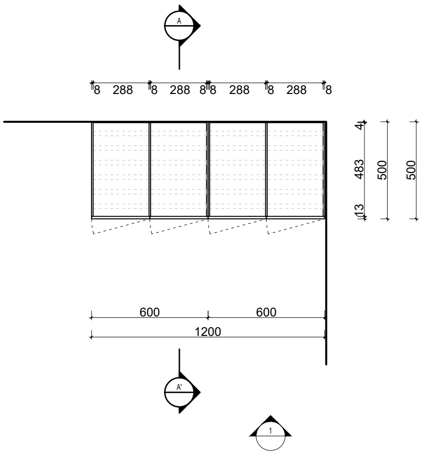
PŮDORYS HORIZONTÁLNÍ ŘEZ 1:20 @ A1
