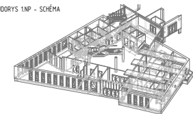
PŮDORYS 1.NP - SCHÉMA
