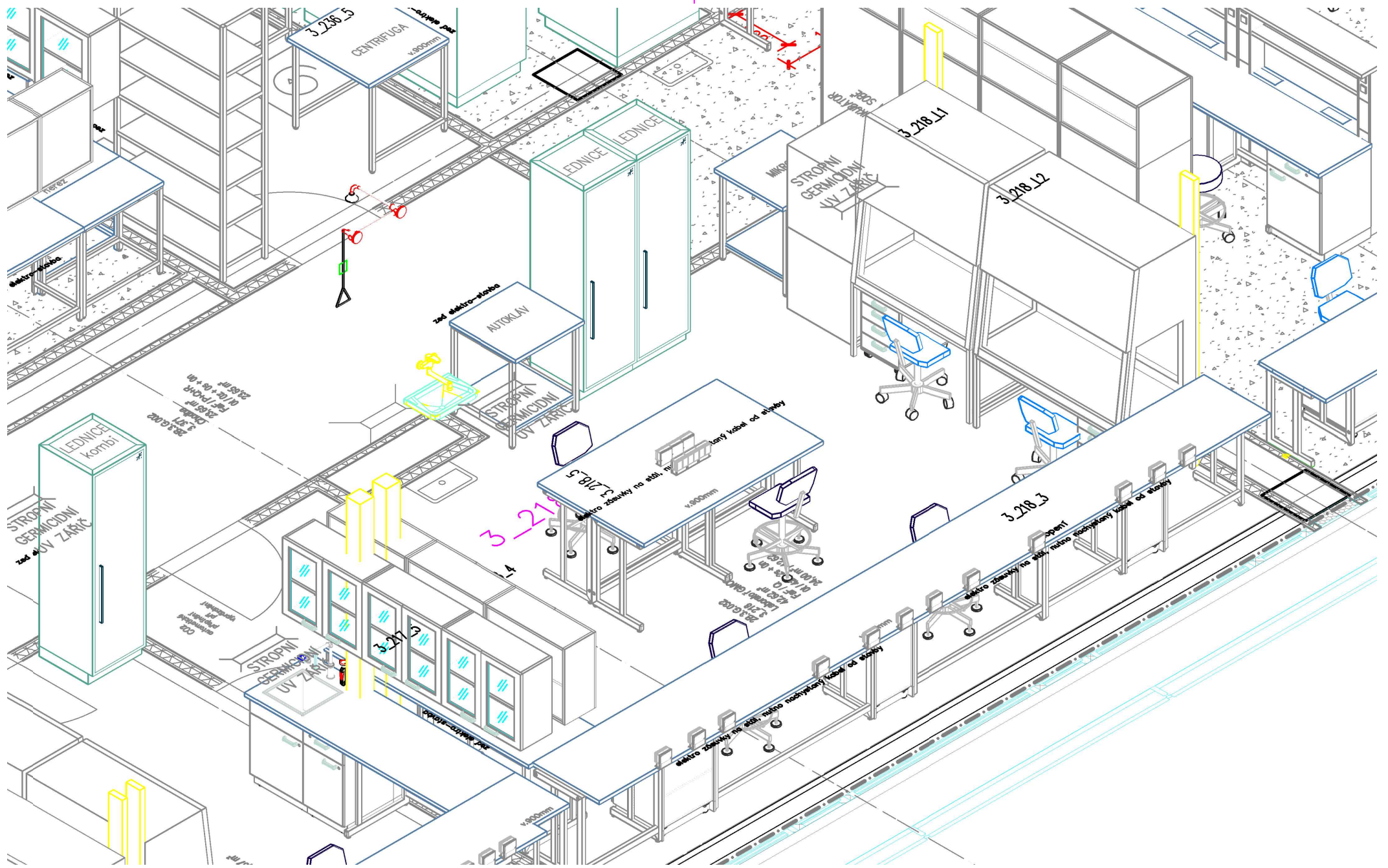
3_218 – pohled 01
