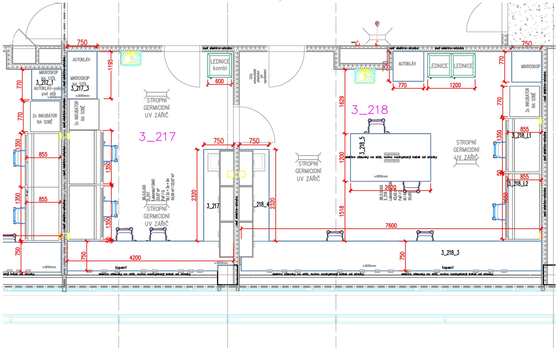
3_217, 3_218 – půdorys
