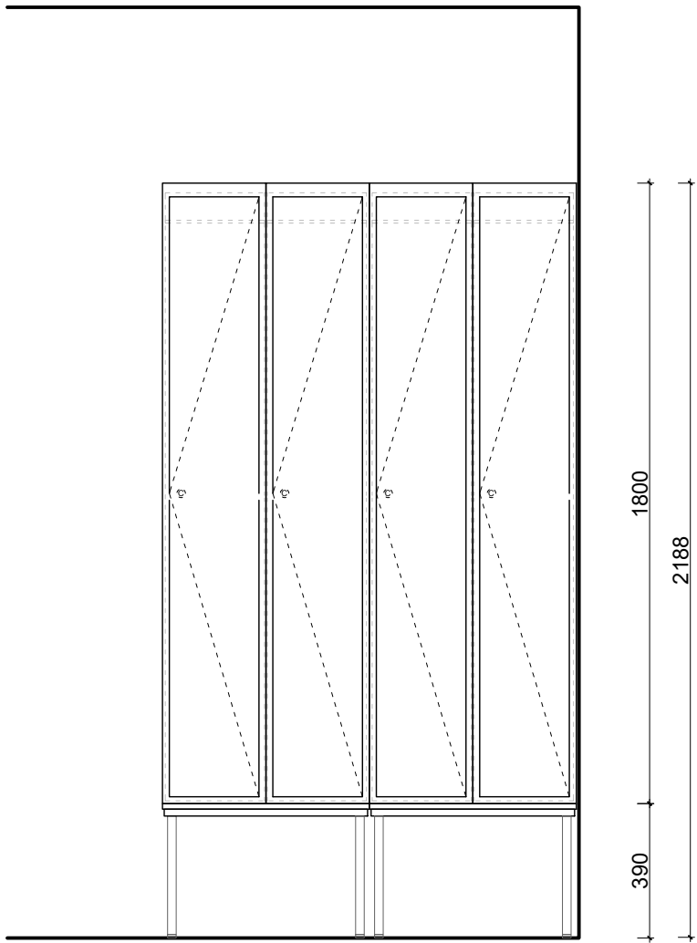
POHLED_1 ČELNÍ 1:20 @ A2
