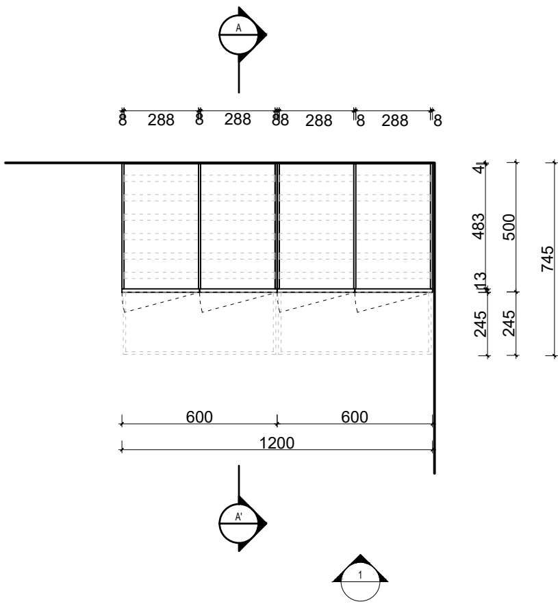
PŮDORYS HORIZONTÁLNÍ ŘEZ 1:20 @ A2
